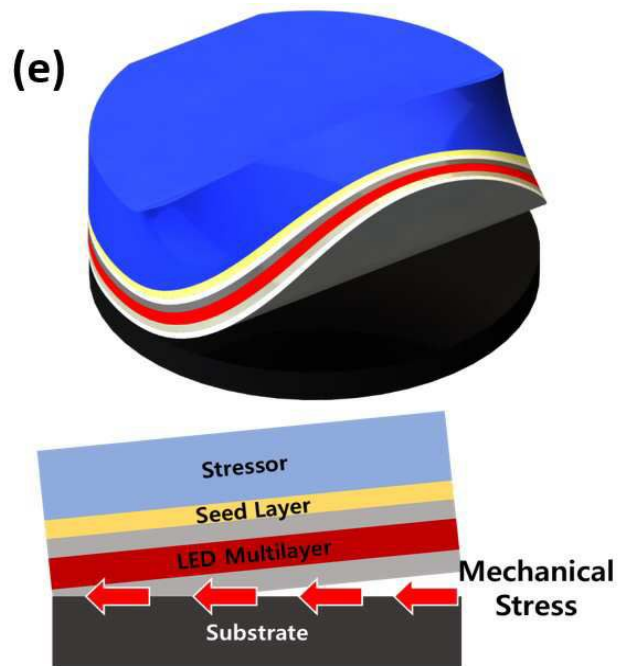
(e) LED Layer Exfoliation by Stressor (응력층의 기계적 스트레스에 의한 LED층 박리)
