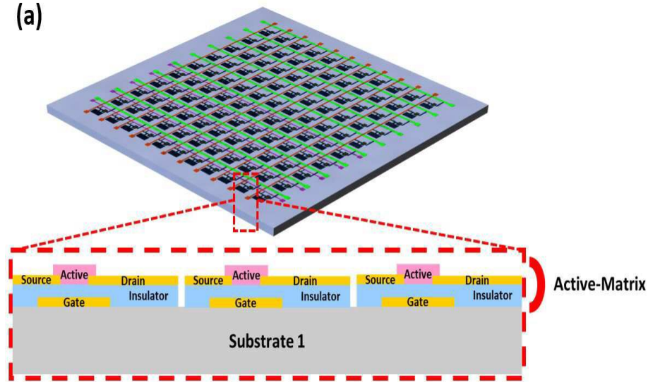
(a) Active-Matrix Backplane on Substrate 1 (제1기판에 디스플레이용 액티브 매트릭스 어레이 형성)
